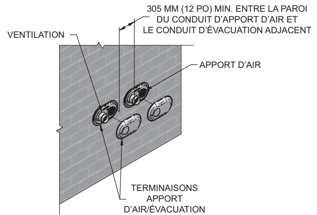
Figure 4-6A Plusieurs terminaisons d'évacuation (doit aussi être conforme à la Figure 4-1A)
