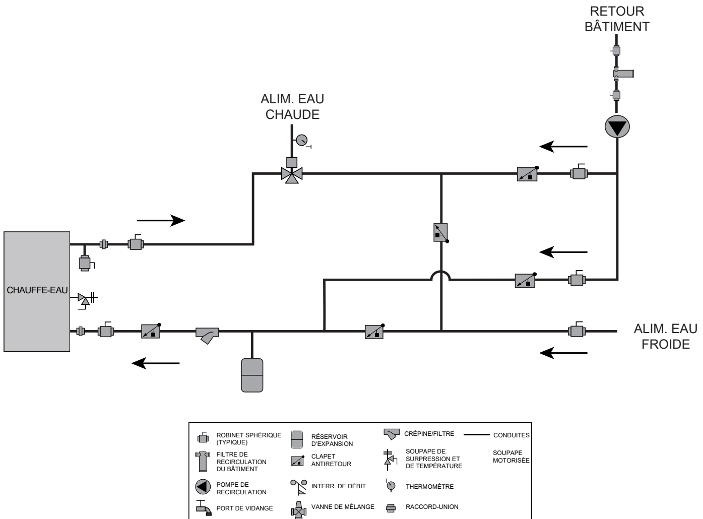
Figure 7-2 Réchauffeur simple - Température unique - Recirculation ECS
