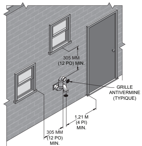
Figure 4-3B Dégagement aux ouvertures du bâtiment en option avec raccords non fournis
