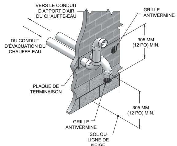
Figure 4-1B Terminaisons d'apport d'air et d'évacuation murales en option en PVC/CPVC (non fournies)
