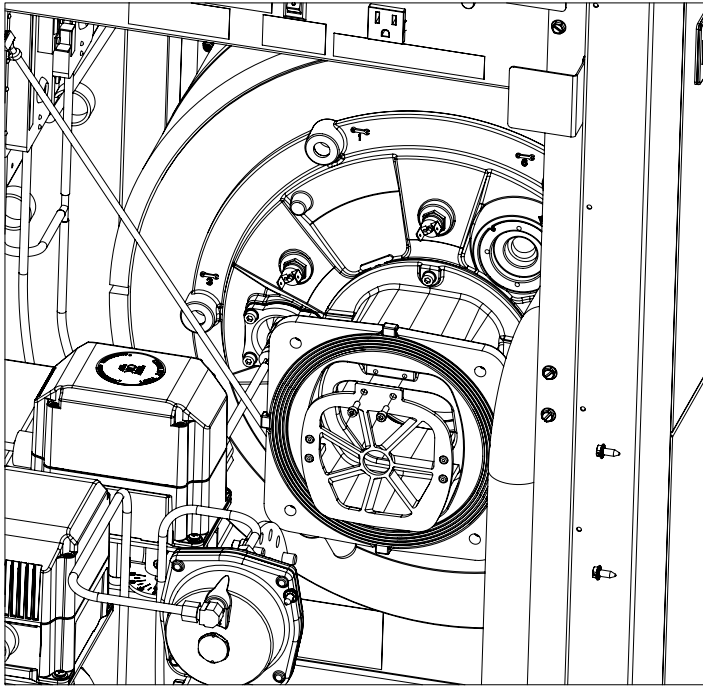
Figure 8-3 Insérez l'obturateur d'air dans le collecteur
