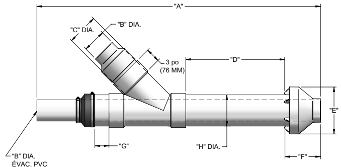
Figure 4-9 Dim. terminaison concentrique d'évacuation – modèle 500
