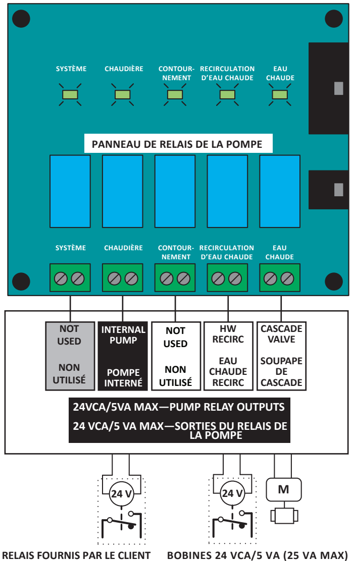
Figure 9-4 Sorties de relais de vanne et de pompe en cascade
