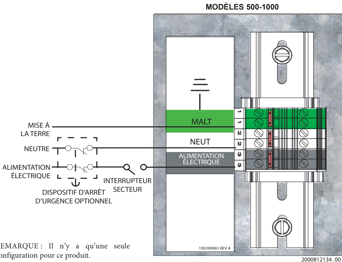
Figure 9-1 Raccordements de tension secteur sur site
