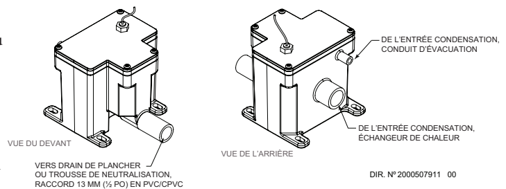
Figure 13-1 Collecteur de condensation
