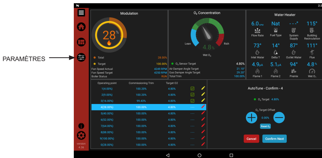
Figure 11-2 Écran de mise en service
