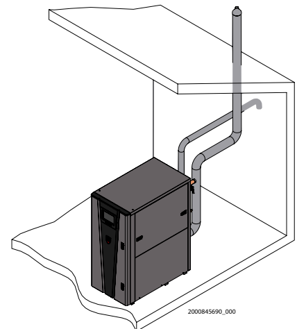
Figure 3-5 Évacuation verticale, apport d'air mural
