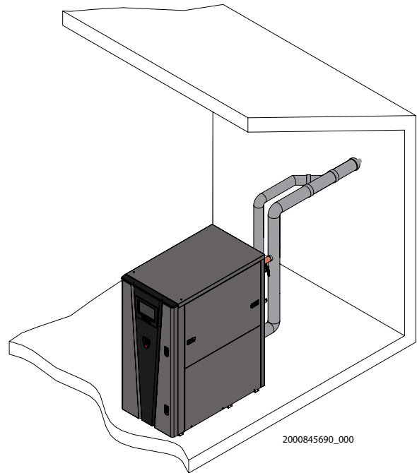
Figure 3-2 Terminaison murale concentrique en PVC/CPVC
