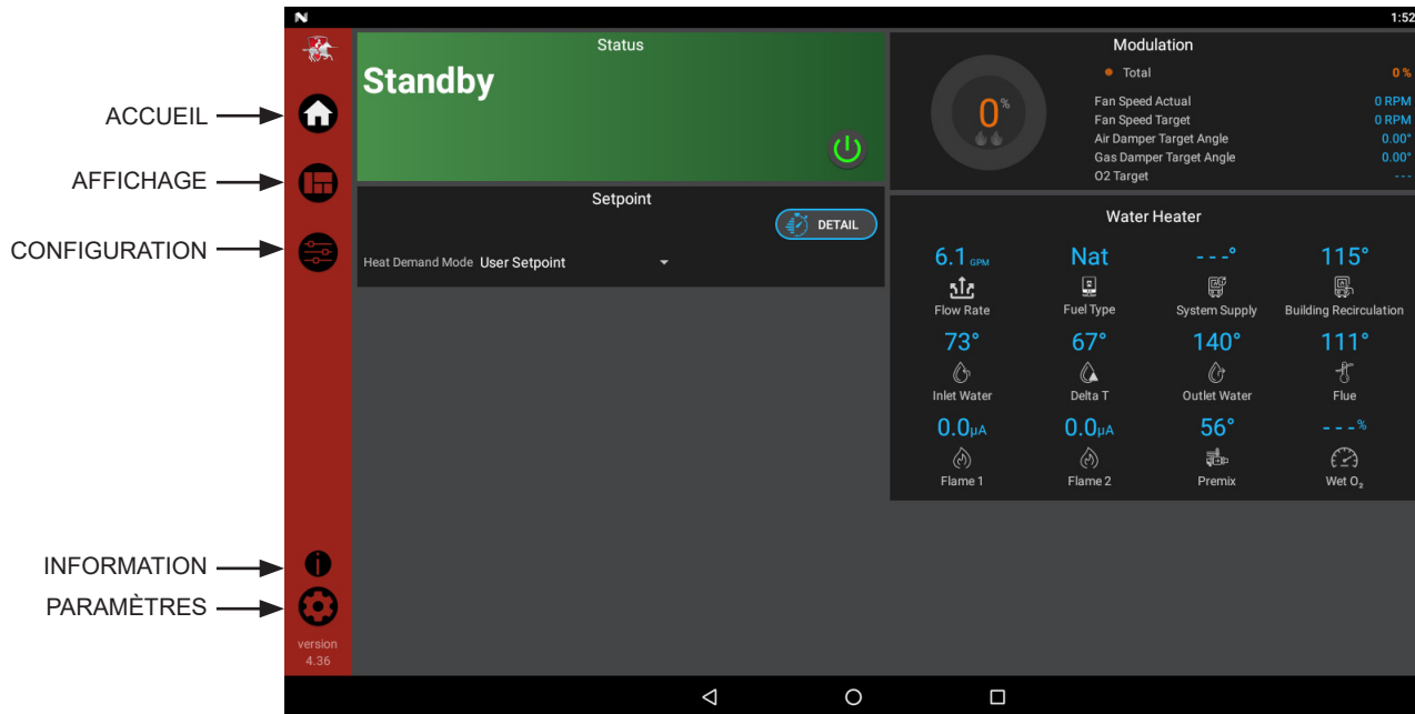
Figure 12-1 Écran d'accueil
