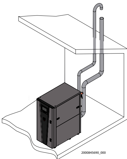
Figure 3-3 Deux conduits, terminaisons verticales
