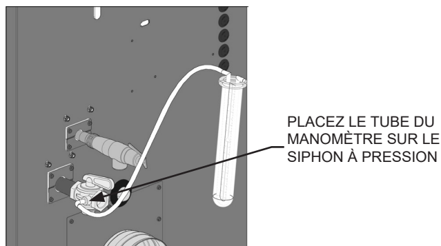
Figure 8-4 Vérification de la pression d'entrée – modèles 500 – 1000
